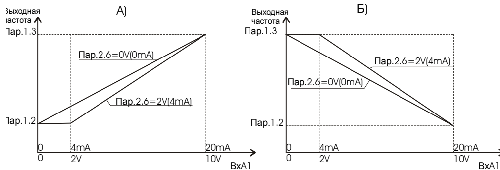
Рис. 7.7 Характеристика управления.
