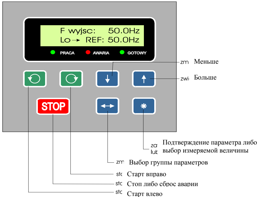
Рис. 5.1 Панель управления.
